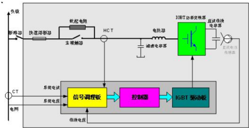
图 2-2 APF 内部控制原理图
