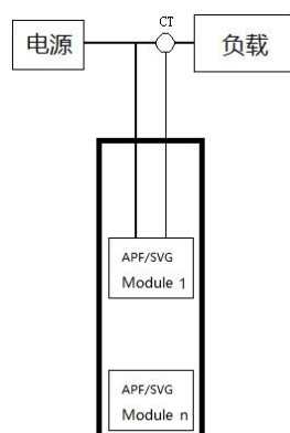
C: 多模块负载侧采样
