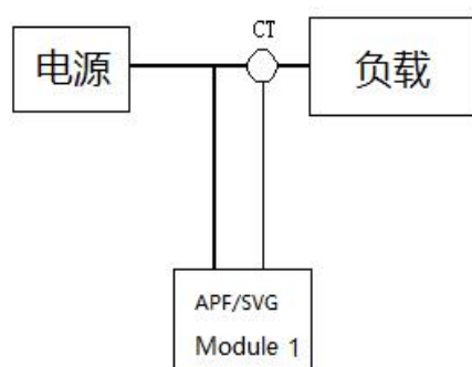
A: 单模块负载侧采样
