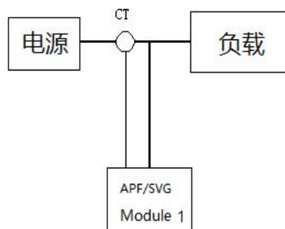
B: 单模块电网侧采样
