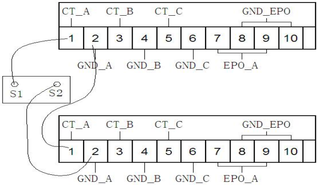
图 4-11 CT 线串联连接示意图
