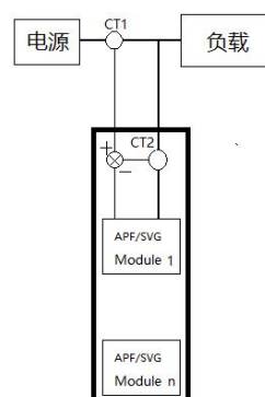
D: 多模块电网侧采样
