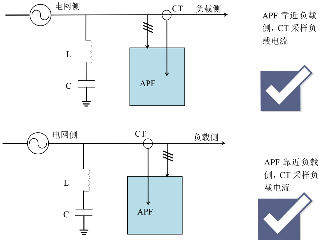
图 4-7 APF 与电容器补偿的位置关系
