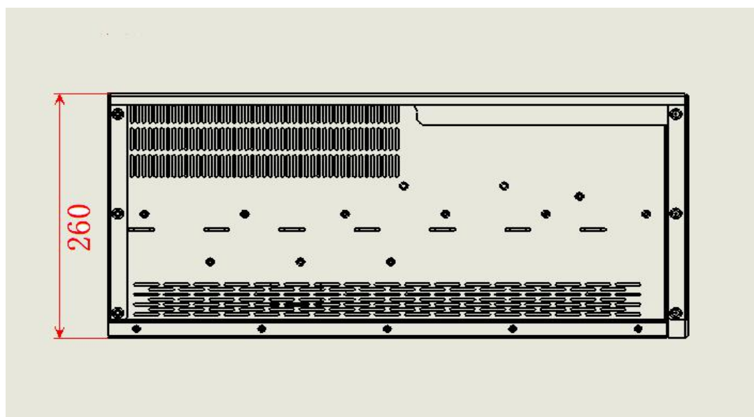
图 4-3 APF 功率模块外形尺寸 (100A)
